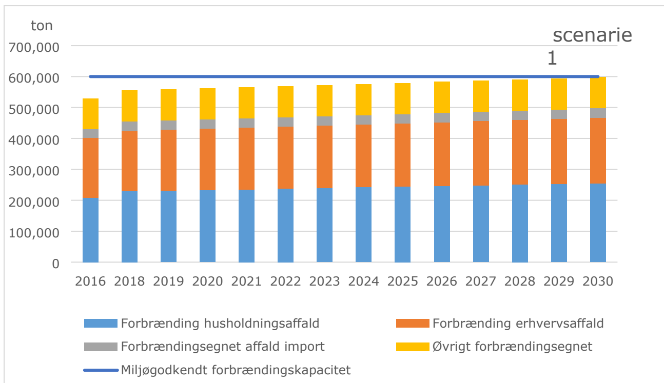
Figur 3: Scenarie 1 - Forbrændingsegneede affaldsmængder og forbrændingskapacitet
